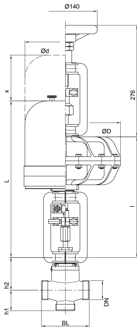
baelz 335 dimensions
