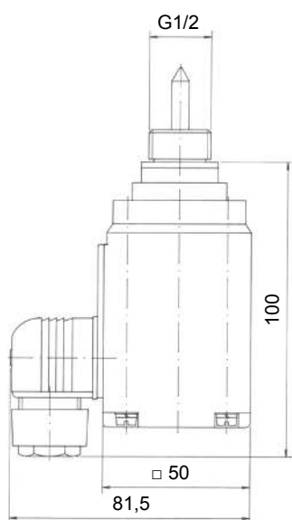
baelz 266st
