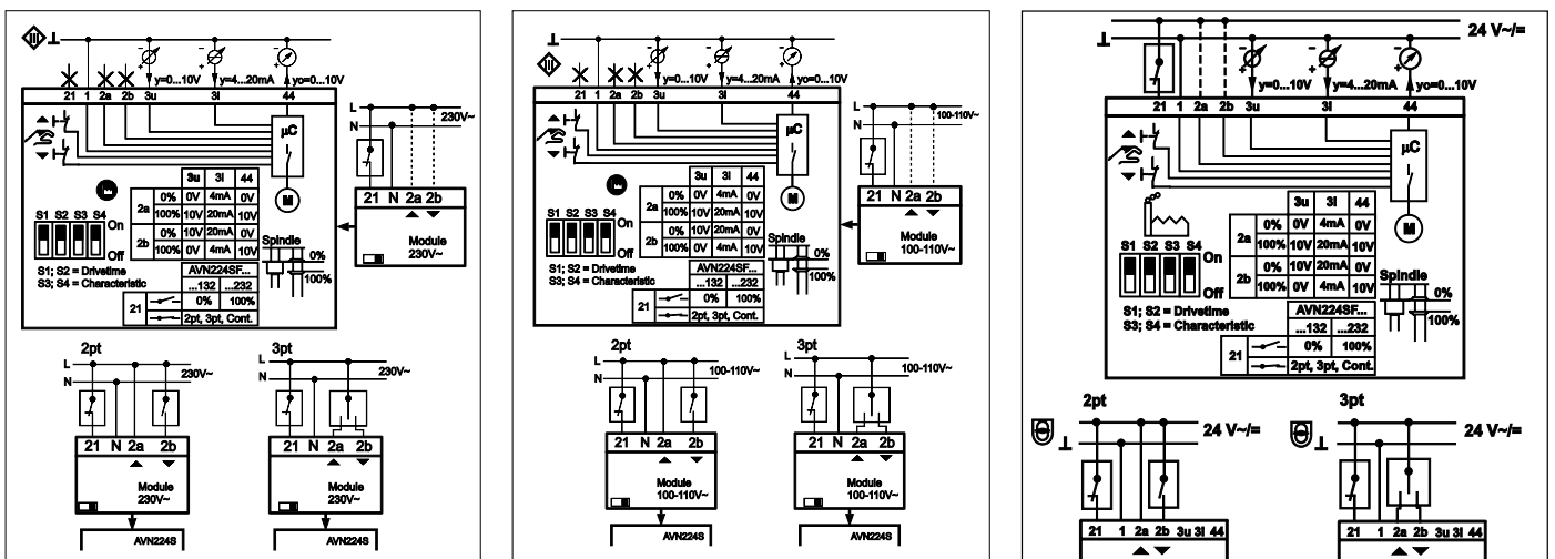
baelz 373-E65 wiring diagrams
