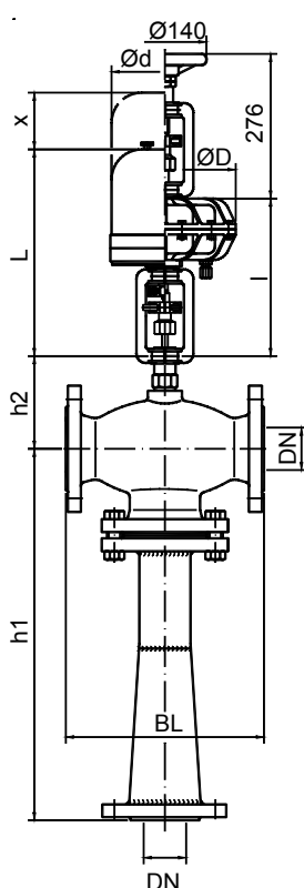
baelz 590 DN15-125
